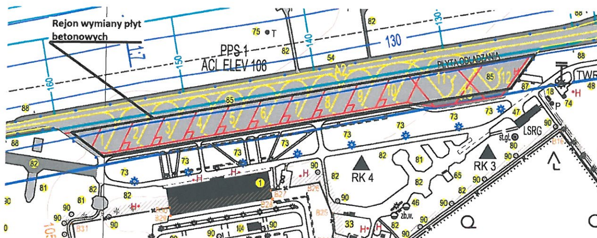
Rys. 3. Schemat usytuowania rejonu prac naprawczych.
